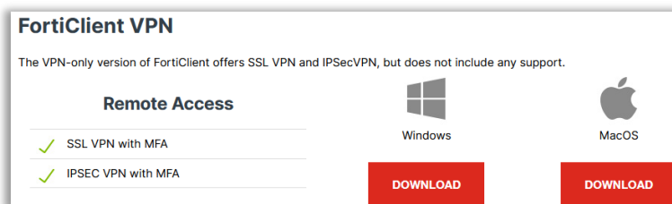
Abbildung 4: FortiClient Download
